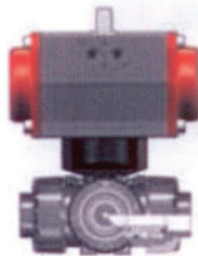
TKD / CP ΤΡΙΟΔΕΣ ΒΑΝΕΣ ΜΕ ΠΛΕΥΜΑΤΙΚΟ ΚΙΝΗΤΗΡΑ DN10/50 PVC-U, PVC-C, PP-H, PVDF
